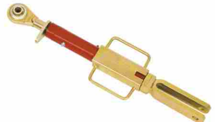
CODE : 109 Leveling Assembly M/F J-Series (N.S.T.) Heavy Duty
